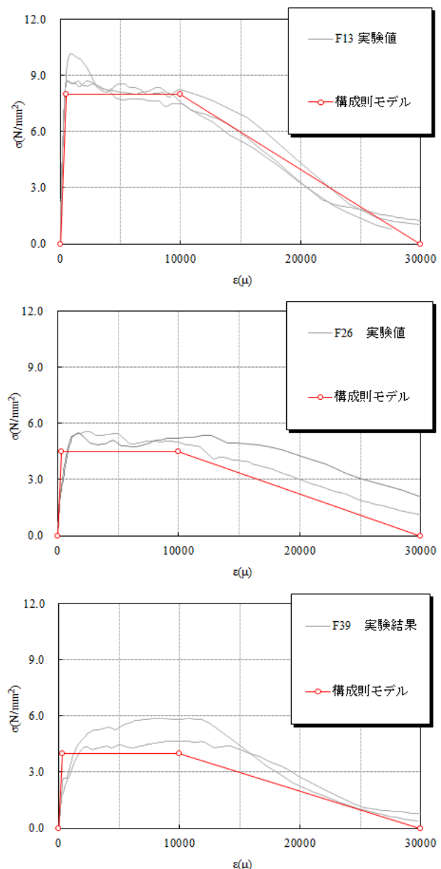
図.2 曲げ強度-下縁ひずみ関係と構成則モデルの比較
