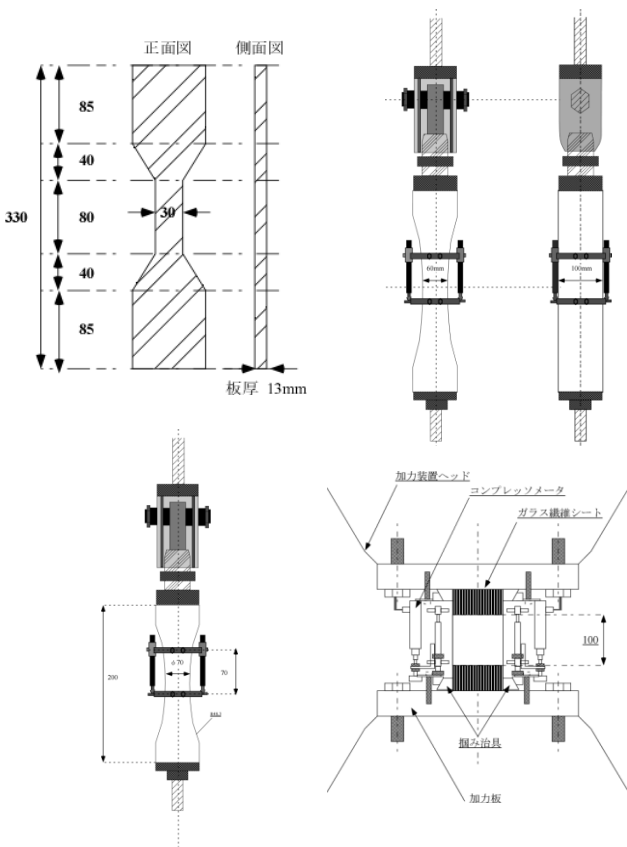
図.1 一軸引張試験 実験方法
